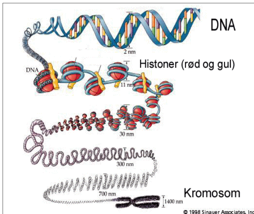
Figur 31 Kromosomstruktur. DNA molekylet komprimeres ved hjælp af kerneproteiner (histoner)
