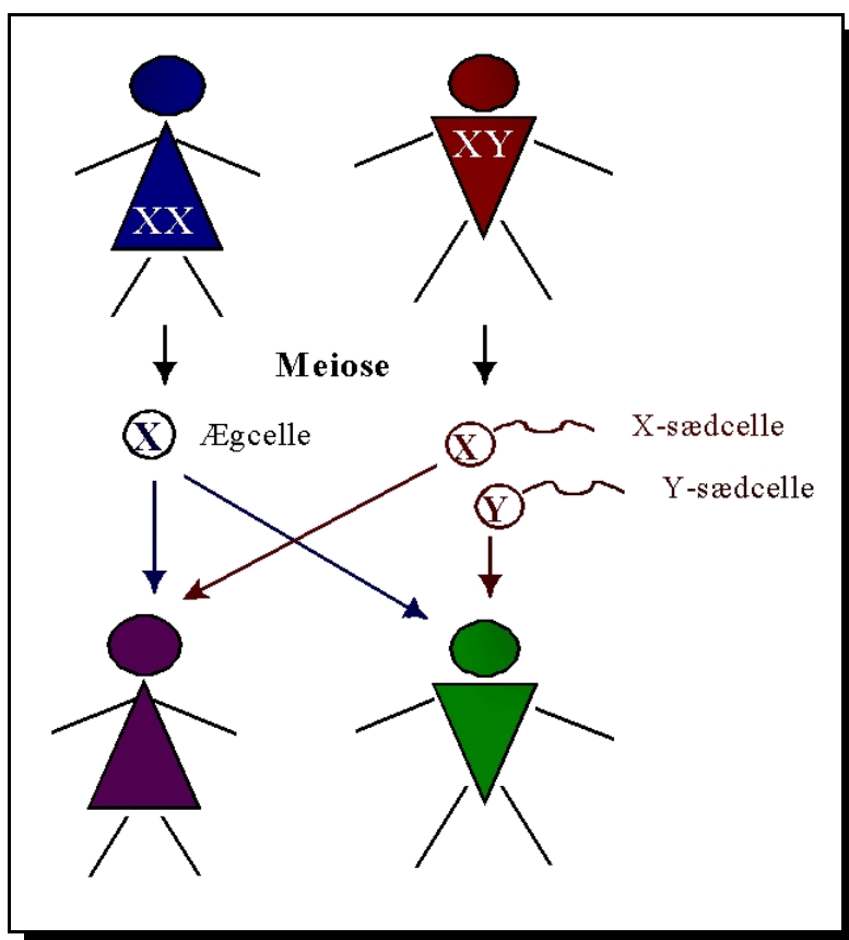
Figur 27 Nedarvning af kønskromosomer
