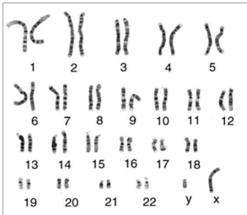
Figur 33 Menneskets 46 kromosomer arrangeret i par efter størrelse. Dette mønster kaldes en karyotype. Der er 22 par autosomer og et par kønskromosomer. Se tabel 38 for en oversigt over gener i de forskellige kromosomer.
