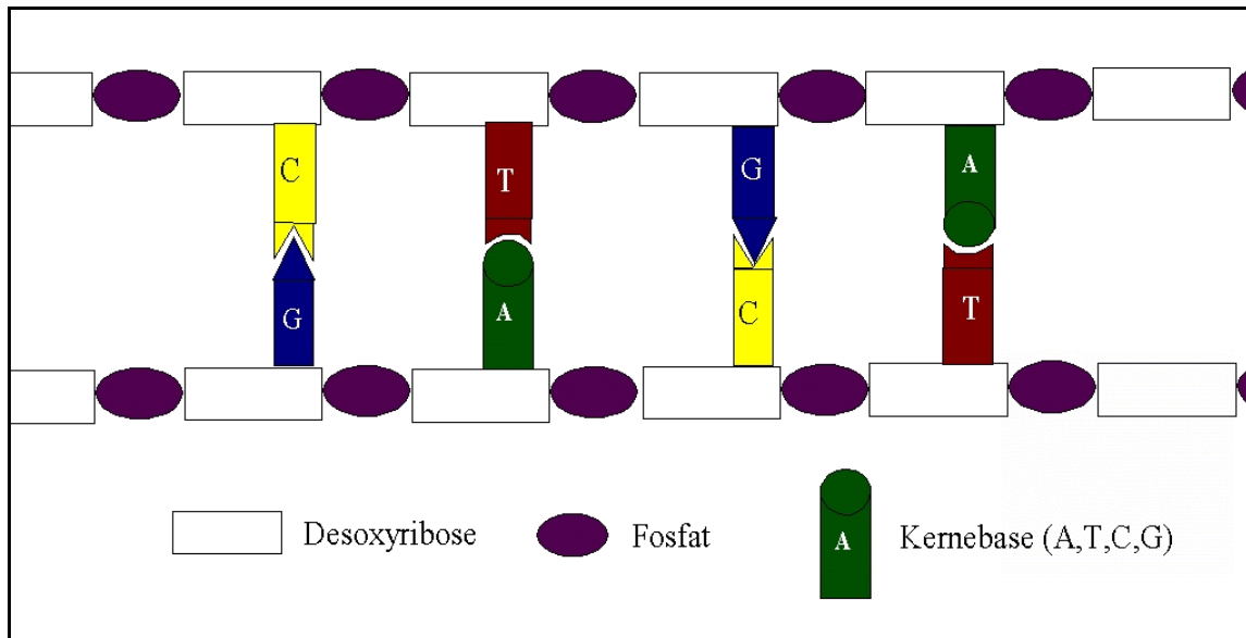
Figur 36 Skematisk oversigt over grundstrukturen i DNA
