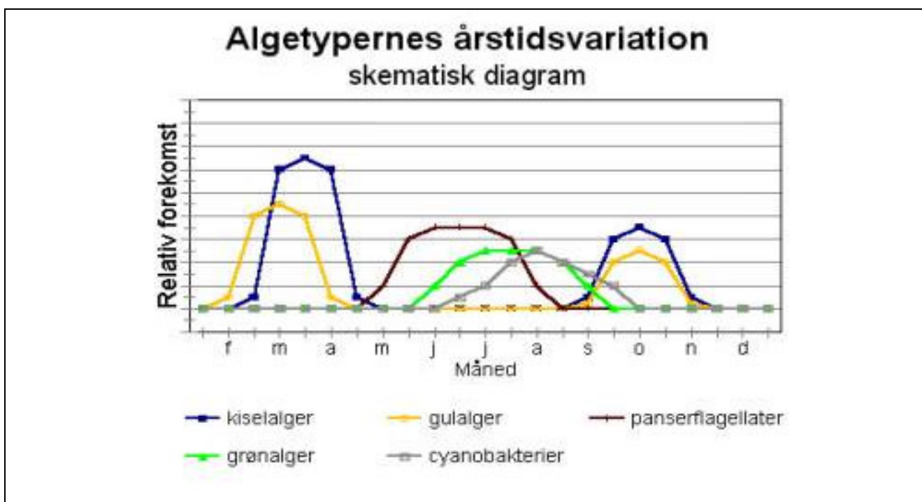
Figuren viser et skematisk og generelt diagram over planktonarternes årstidsvariation.
