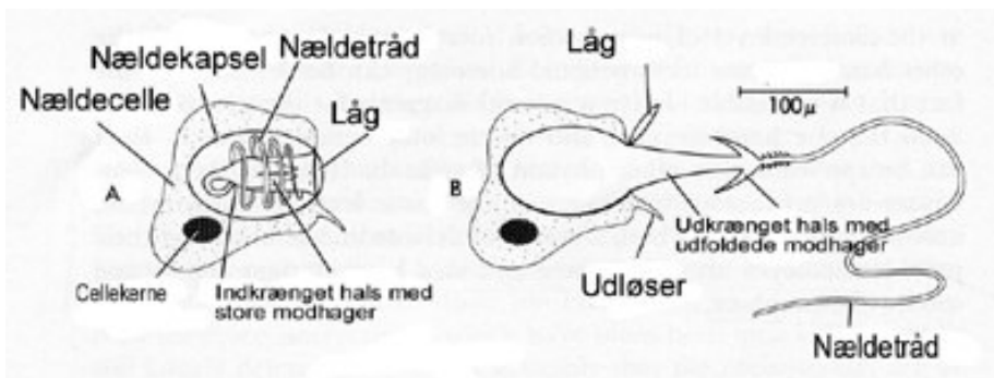
Skematisk tegning af en nældekapsel før (A) og efter udløsning (B).
